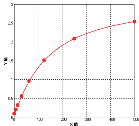
小鼠 EGF 参考标准曲线
