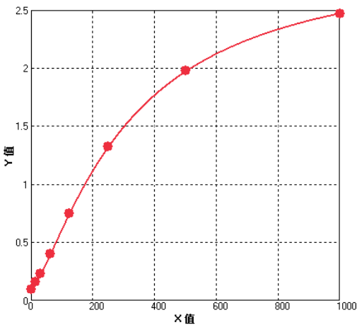
小鼠BMP-9参考标准曲线
